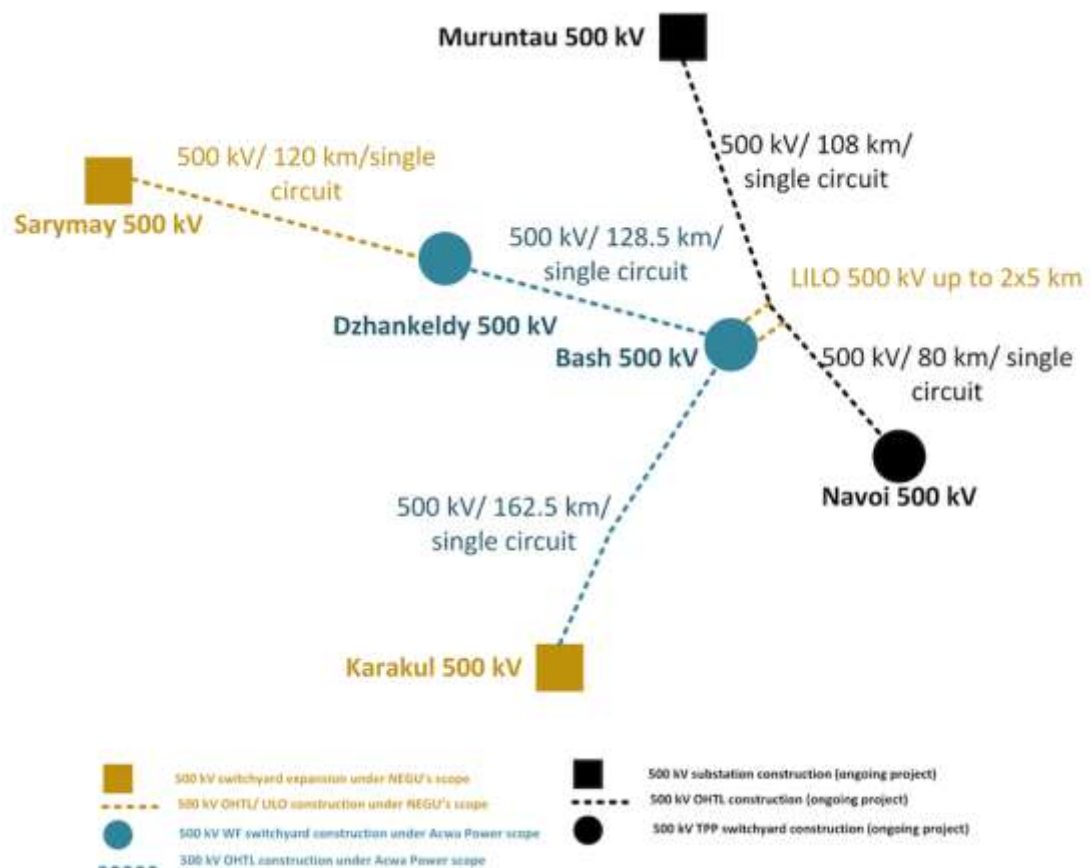
Фигура2-4 Вариант подключения к сети для ветряных электростанций мощностью 1 ГВт АСВА (Джангельды и Баш)
