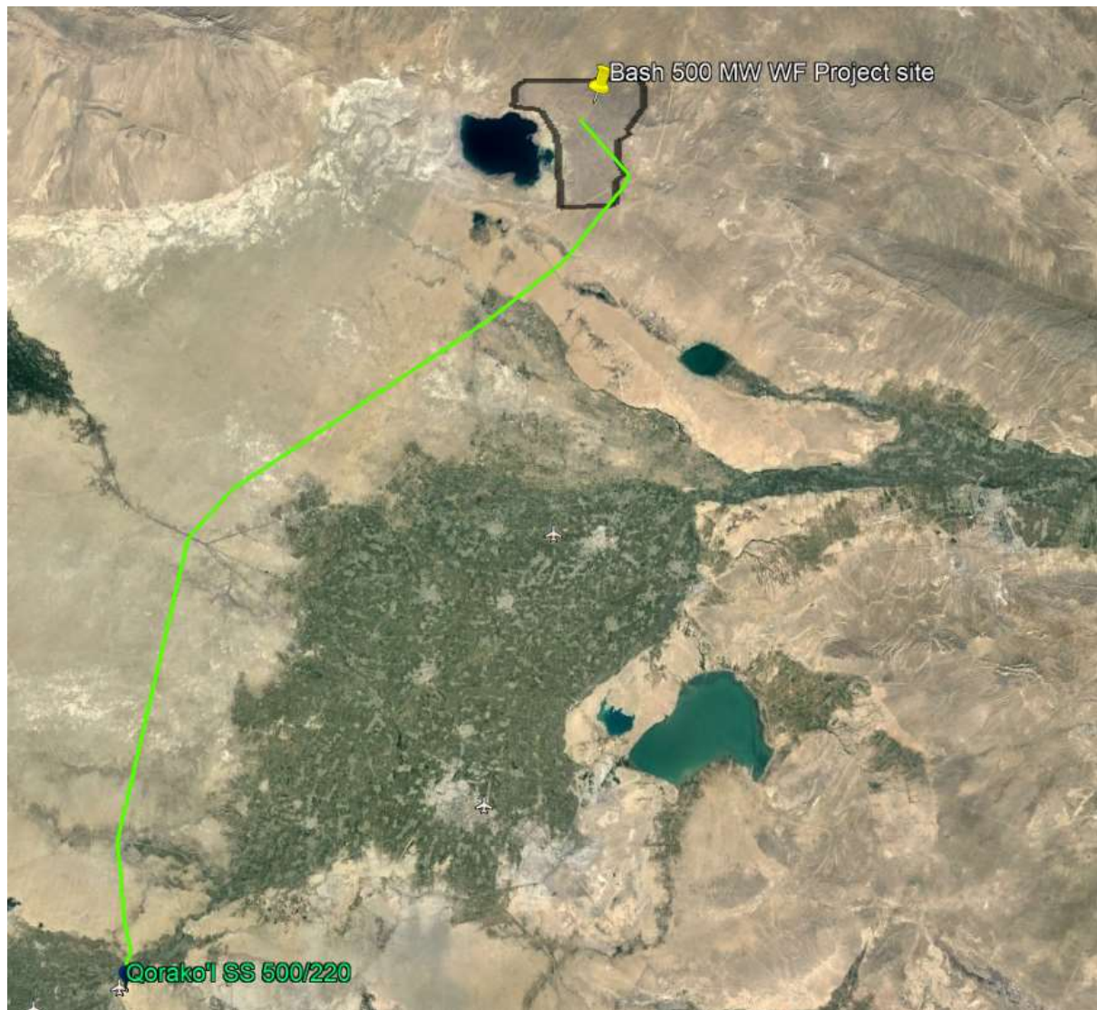
Рисунок 2-2. Схема расположения ВЛЭП протяженностью 162 км от ветряной электростанции Баш до подстанции Каракуль
